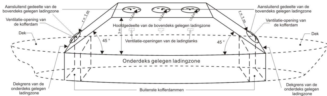
Bovendeks gelegen ladingzone voor diverse tankschepen
