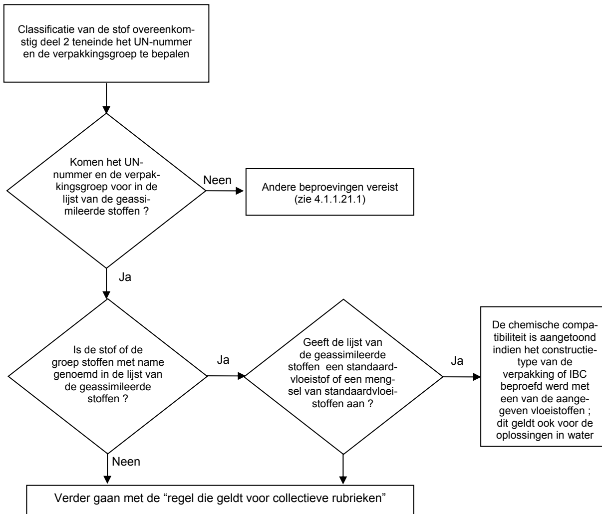
Afbeelding 4.1.1.21.1 : Schema voor het assimileren van de vulstoffen met de standaardvloeistoffen
