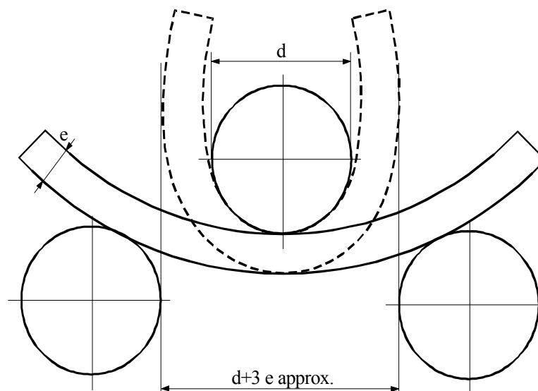
Buigproef
