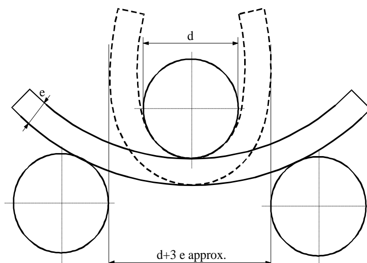
Buigproef
