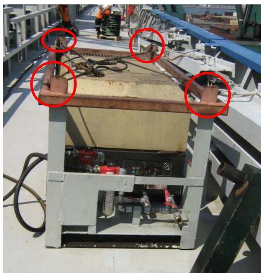
Compressor met 4 aanslagpunten
